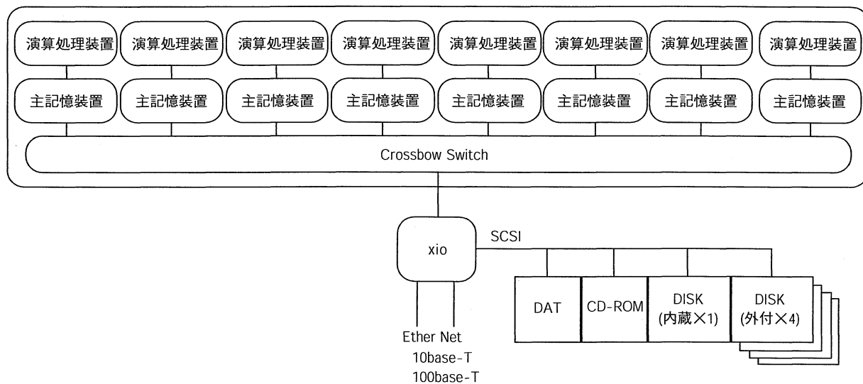
図 3.1.6 NUMA(Non-Uniform Memory Access)型計算機システム
