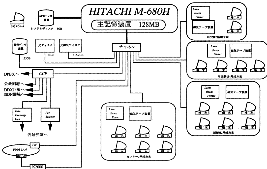
図3.1.1a 大型汎用計算機システム
